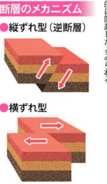
断層のメカニズム
